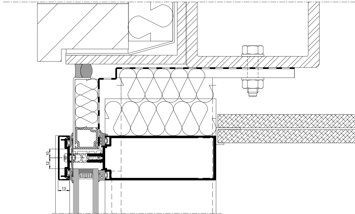
H1 12.01
