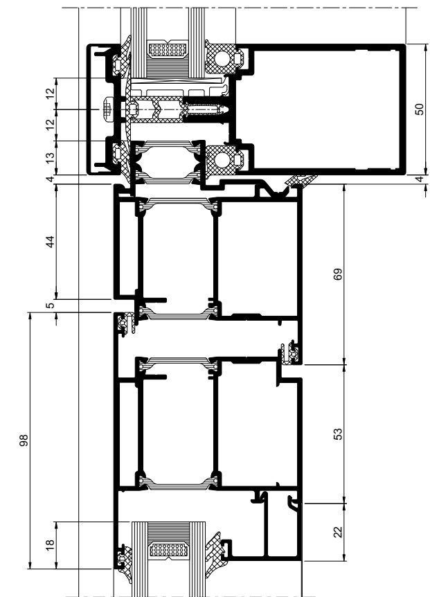
H3 09.01
