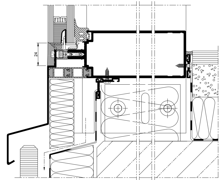
H 06.01
