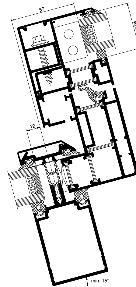
H2 17.01
